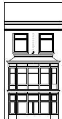
GEVEL MAASBOULEVARD
